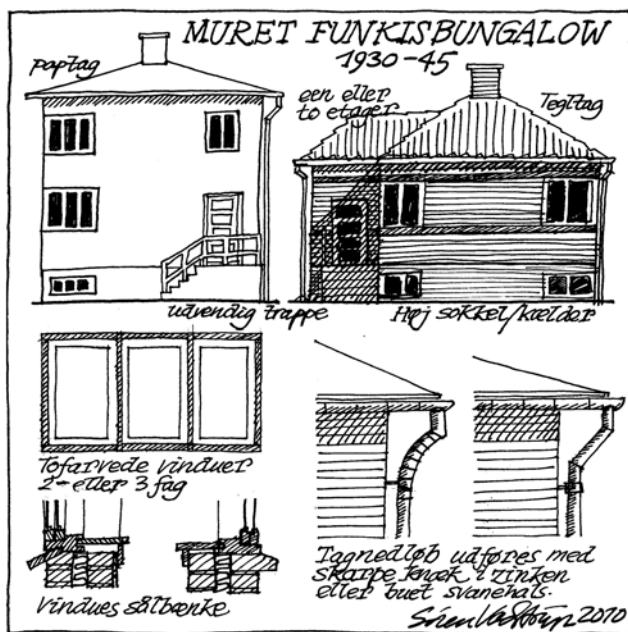
Bygningstypologi-tegning for en muret 'Funkisbungalow', der kombineret med ny-SAVE-Metoden, kan forenkle udpegningen af bevaringsværdige bygninger. Tegning: Søren Vadstrup.
