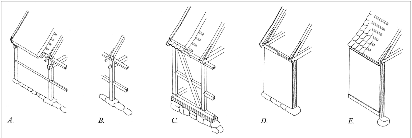
A: Styrtrumskonstruktion med glammede bjælker. B: Styrtrumskonstruktion med gennemstukne bjælker. C: Bindingsværkshus med spærfagskonstruktion. D: Grundmuret vægkonstruktion med saggjel og sternbræt. E: Grundmuret vægkonstruktion med muret og pudset (trukket) hovedgesims.
