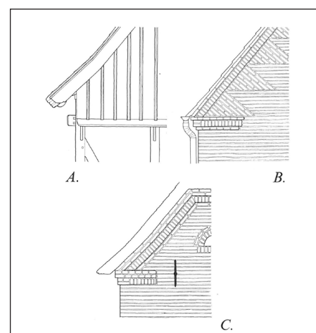
A: Gavlbeklædning af ru eller høvede brædder med affasede dækklister. Beklædningen er formeden afsluttet med vandbræt på trækonsoller. Gavlhængiet er afsluttet med vindskede sommet på lægteenderne, der bærer stråtaget. B: Muret gavlbeklædning med såkaldte strømskifter ved afslutning mod tagkanten, der især fandt vid udbredelse i det murede byggeri omkring 1900. C: Vestjysk muret gavlbeklædning. Hovedgesimsen på facaderne går med rundt om gavlen og fortsætter langs det halvvalmede tag.
