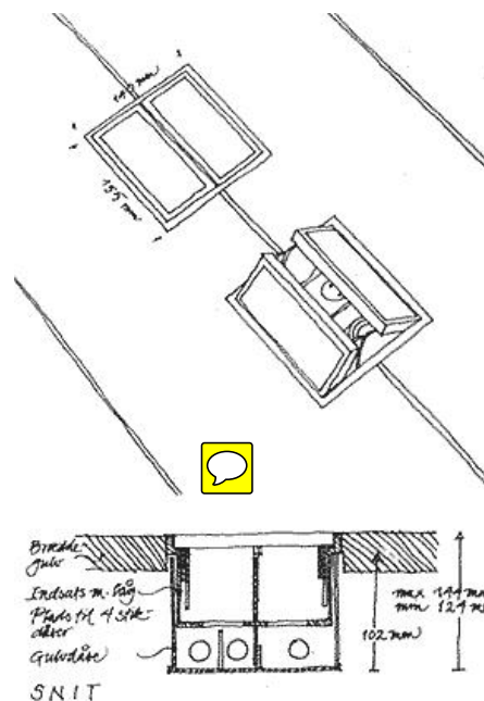
Placering af gulvstikkontakt i gulv.
