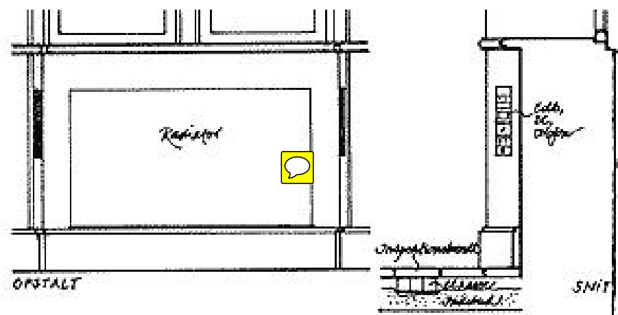
Fremføring af installation under gulv. Udtag er placeret i vindueslysningens glatte panel.
