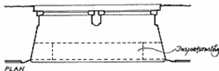
Fremføring af installation under gulv. Udtag er placeret i vindueslysningens glatte panel.
