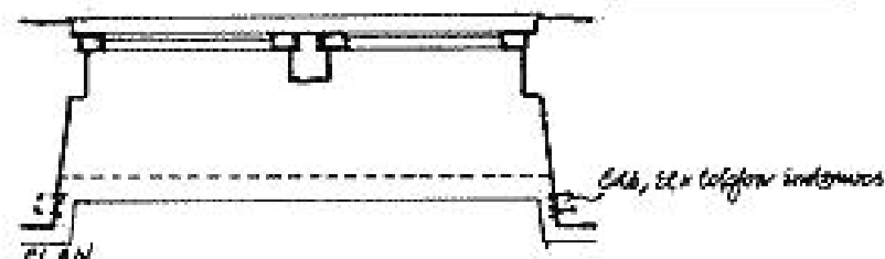
Fremføring af installation gennem murpiller. Fodpanelrepos i vinduesniche med udtag i front og inspektionslås i top.
