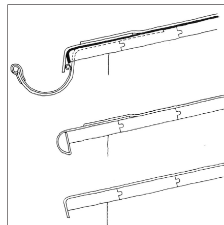
Tre eksempler på traditionelle udhæng til paptaget. Bemærk at rendejernene er nedstemt i bræddeunderlaget. De to nederste eksempler er med enkeltinddækning.
