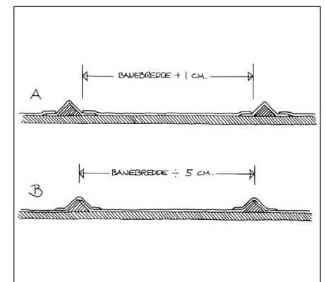
To metoder for listedækning - B er den klassiske metode.
