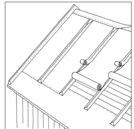
Principtegning for det traditionelle, listedækkede paptag.
