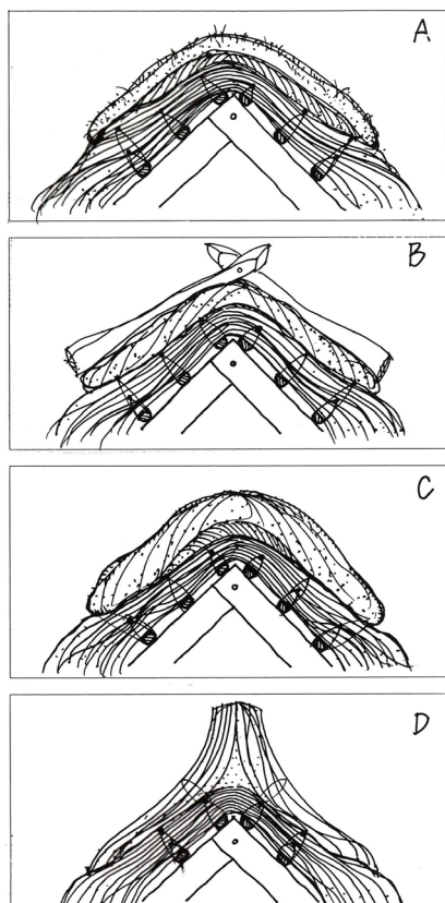
Forskellige mønningstyper A: Mønning med tørv. B: Mønning med kragetræer. C: Mønning med halm eller lyng, fastholdt med galvaniseret net. D: Holstensch mønning.
