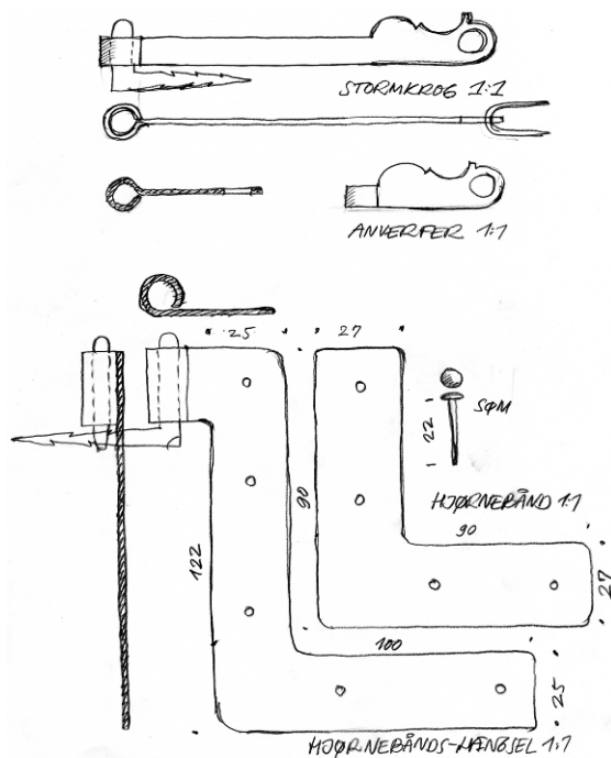
WADSTRUP VIBY BYGADE 12, st. Viby VINDUESBESLÅG 1:1 Søren Vadstrup marts 05
